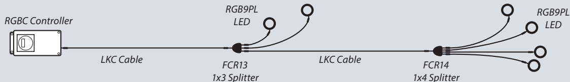
Cable LKC5030
